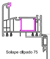
Marco estándar Hoja balconera (perfil vierteaguas)
