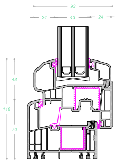
Marco estándar Hoja de ventana
