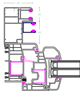
Guía persiana 158 mm
