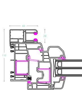
Guía persiana 110 mm
