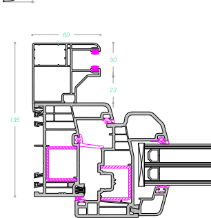
Guía persiana 135 mm
