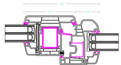
Nudo fijo-hoja reforzado
