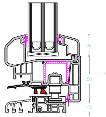
Umbral aluminio Hoja ventana
