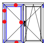
Hoja pasiva. Palanca rebajo. punto cierre superior/interior/lateral
