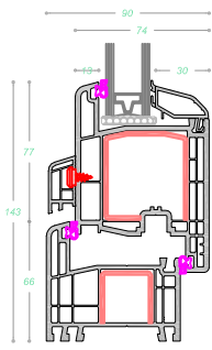
Marco estándar Hoja balconera (perfil vierteaguas)
