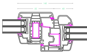
Nudo fijo-hoja
