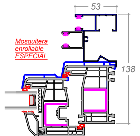
G7 Profundidad 138 mm
