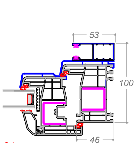
G4 Profundidad 100 mm
