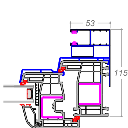
G5 Profundidad 115 mm
