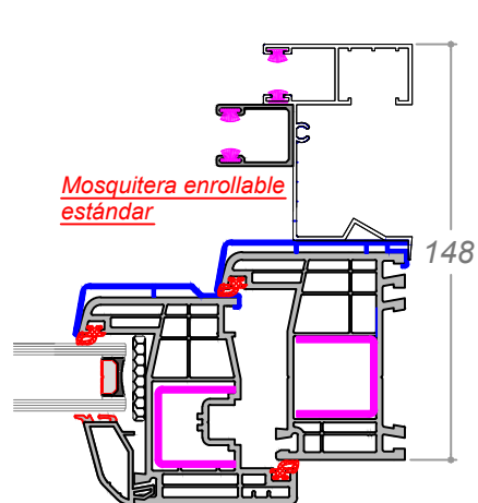
G8 Profundidad 148 mm (motor)
