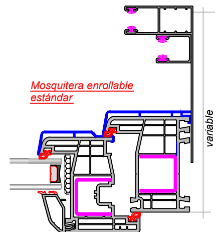
G9 Profundidad variable (motor)
