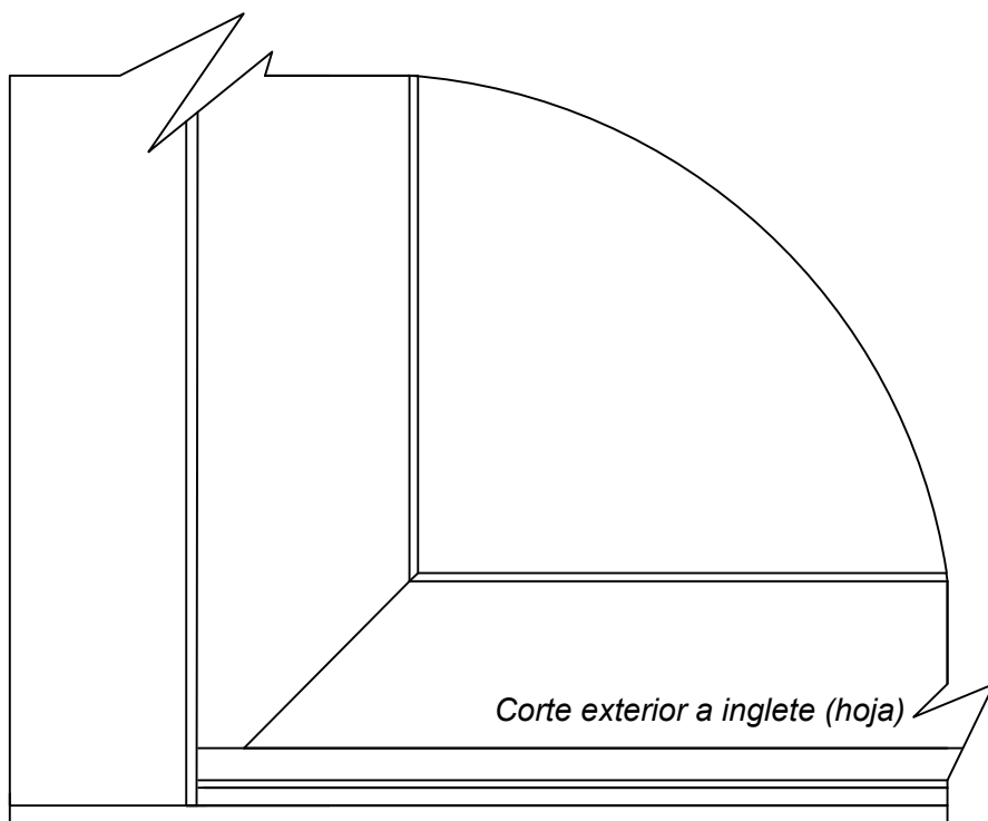
Seccion corte pvc + aluclip PUERTA de calle UMBRAL INFERIOR
