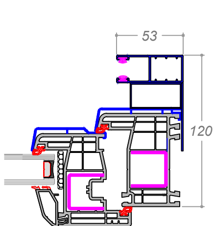
G6 Profundidad 120 mm
