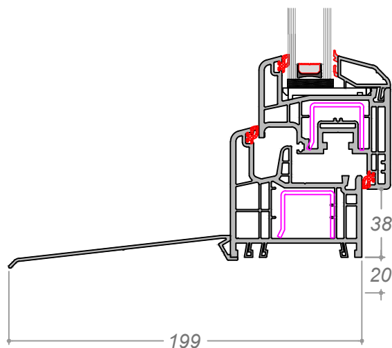
Vierteaguas Aluminio 125 mm P25
