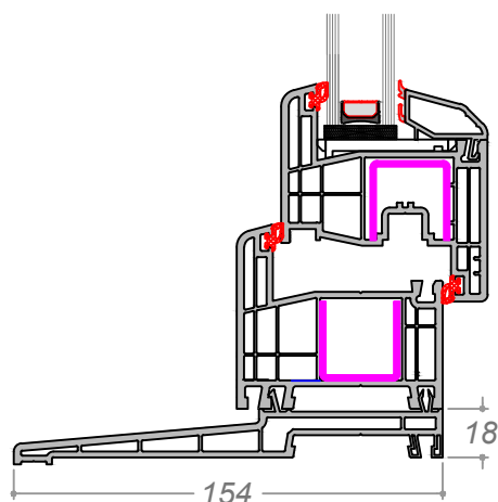
Vierteaguas Pvc 150 mm P26
