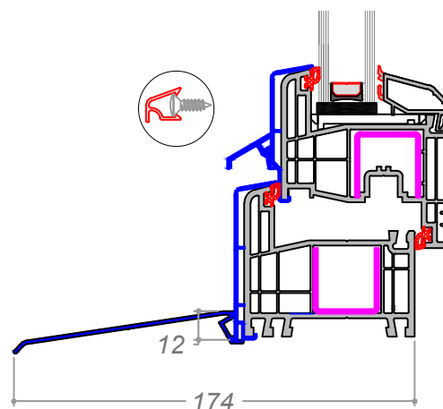
Vierteaguas aluminio 96 mm en aluclip P24
