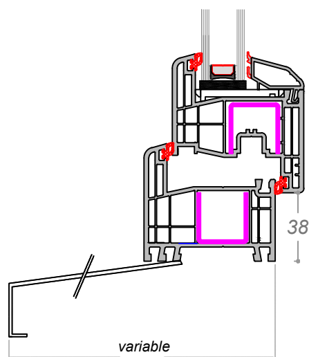
Vierteaguas chapa aluminio variable P27
