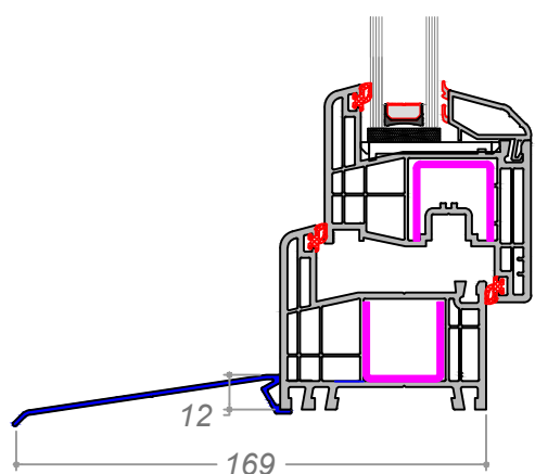
Vierteaguas aluminio 96 mm P24
