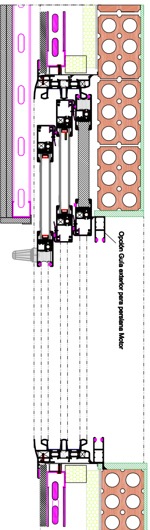
SECCIÓN HORIZONTAL ABIERTA
