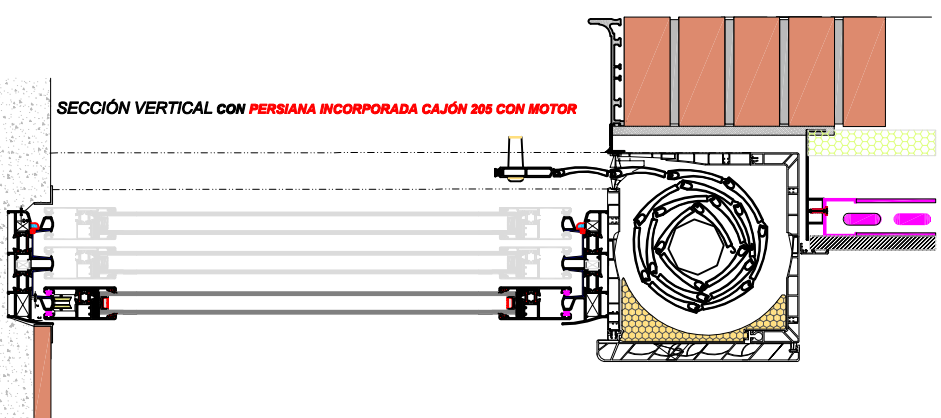
SECCIÓN VERTICAL sin PERSIANA
