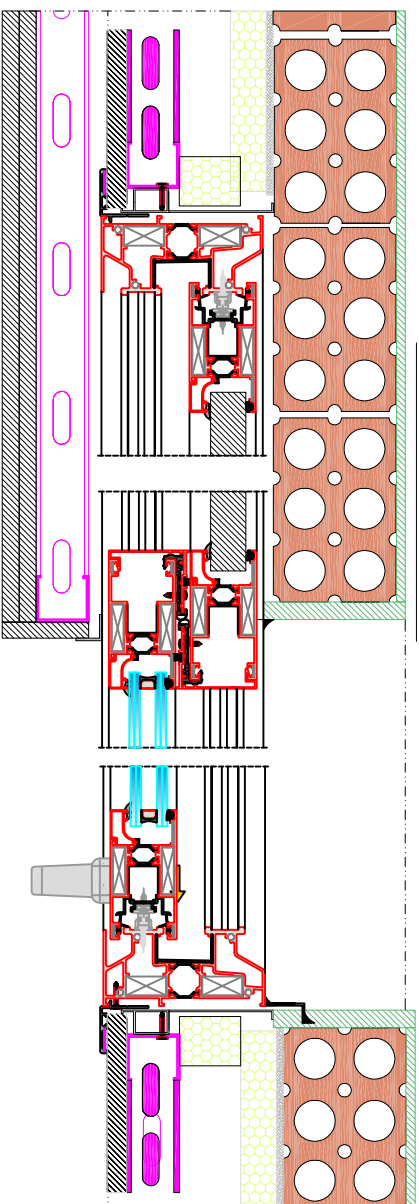
SECCIÓN HORIZONTAL POSICIÓN CERRADA
